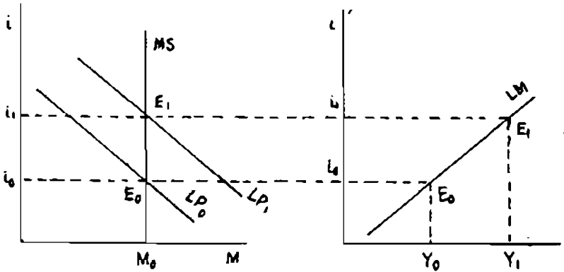
Hình 5.6: đường LM
