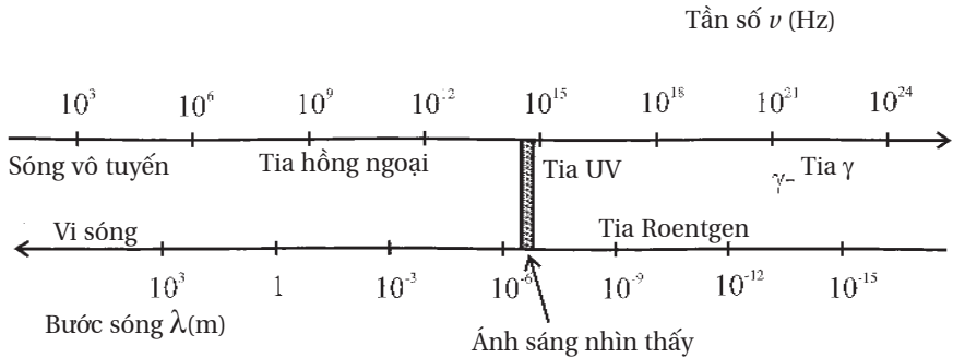
Hình 1.3. Phổ bức xạ điện từ, xác định cho cả tần số \nu và bước sóng \lambda .
