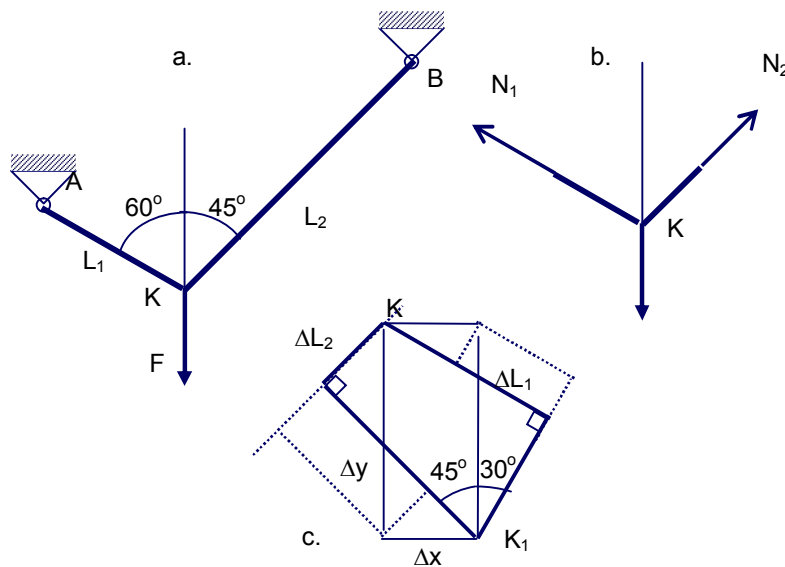
Hình 5.6. Ví dụ tìm dịch chuyển các điểm của hệ thanh liên kết khớp
