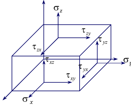
Hình 2.3. Thành phần ứng suất tại phân tử
