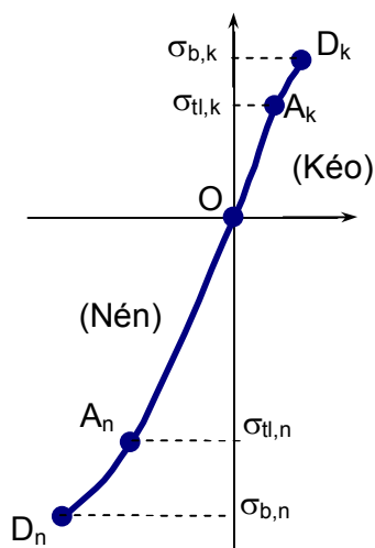
Hình 3.5. Quan hệ ứng suất – biến dạng trong thí nghiệm kéo và nén vật liệu dẻo
