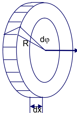
Hình 6.4. Biến dạng của phân tử thanh chịu xoắn
