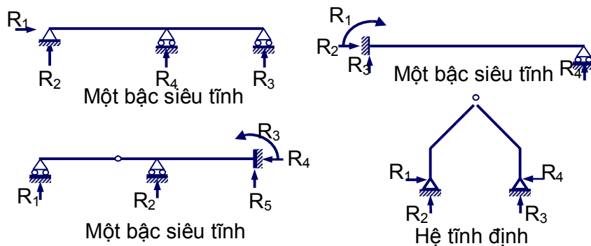
Hình 10.1. Các ví dụ về bậc siêu tĩnh nội
