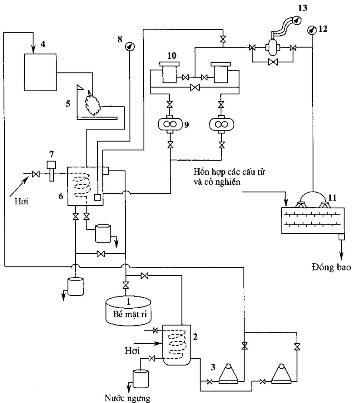
Hình 234. Sơ đồ dây chuyền chuẩn bị mật rì và trộn vào thức ăn hỗn hợp:
