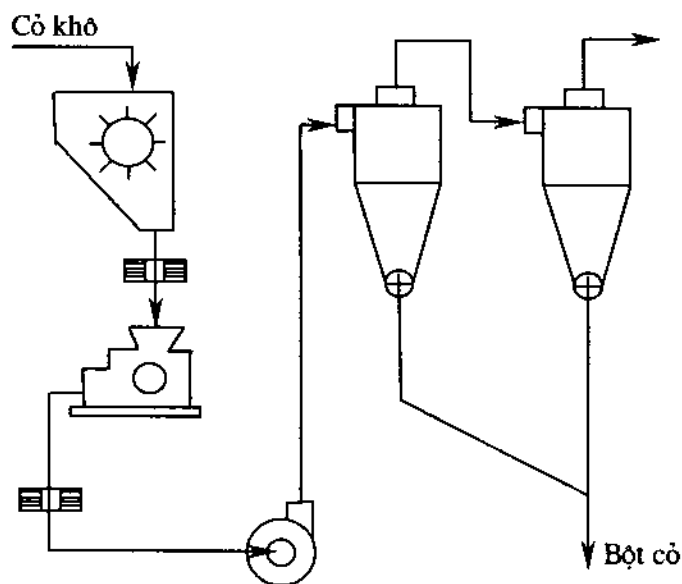
Hình 228. Sơ đồ nghiền cò khô.
