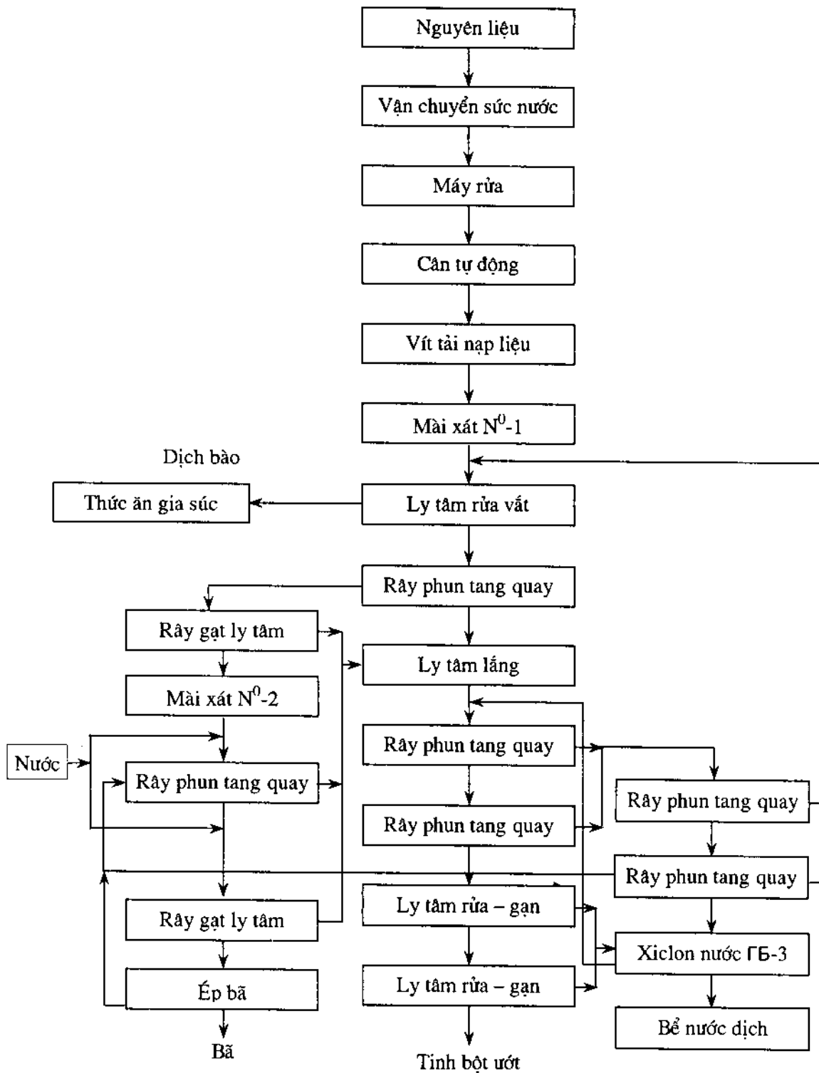
Hình 193. Sơ đồ dùng máy ly tâm rửa gan.
