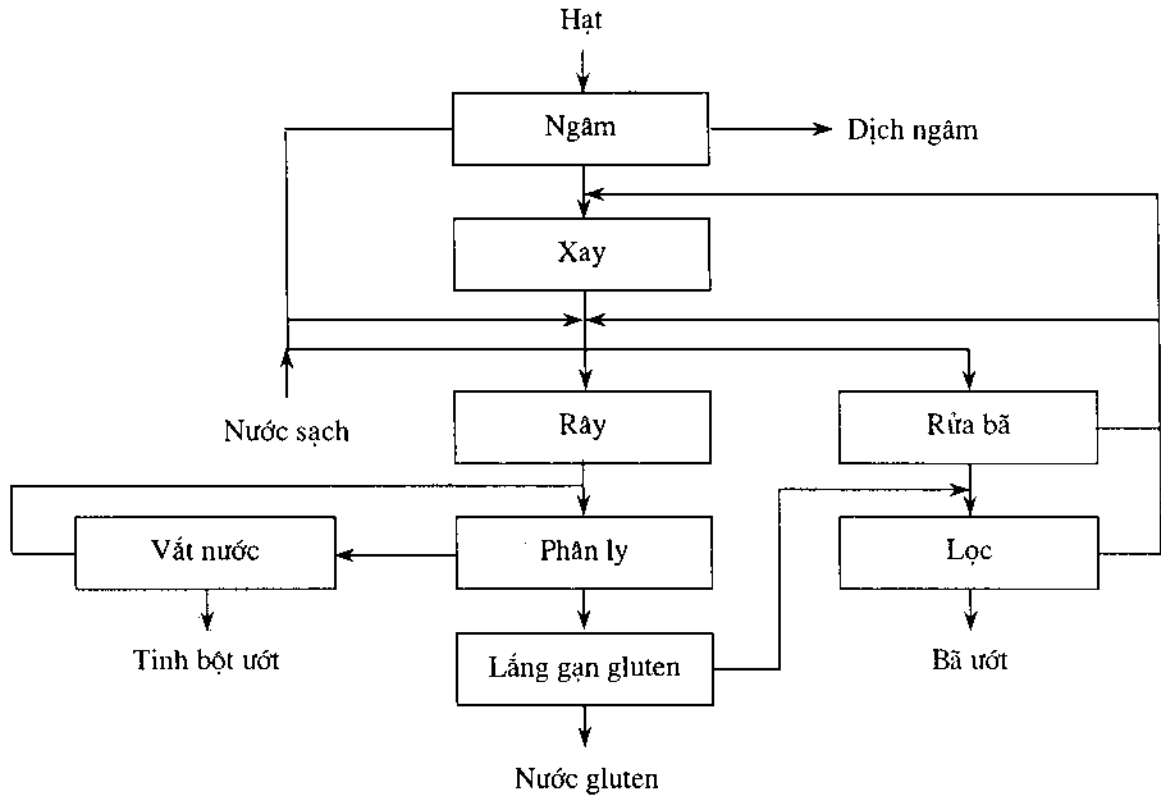
Hình 201. Sơ đồ thu gọn cho xí nghiệp năng suất thấp.
