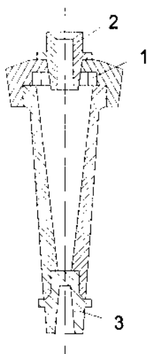
Hình 191. Xi-clon nước đơn.
