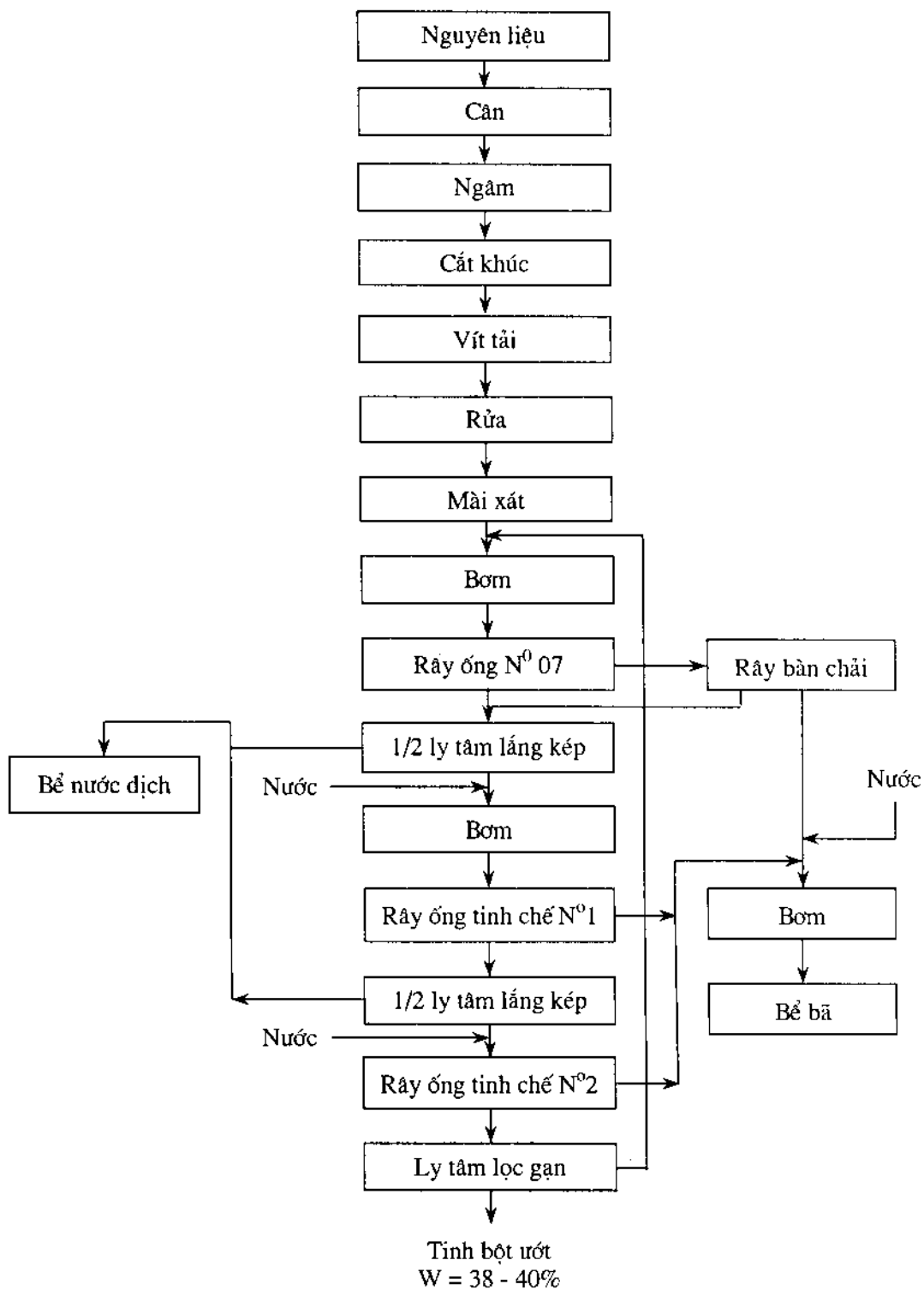
Hình 196. Sơ đồ công nghệ sản xuất tinh bột sắn bằng máy АПЦ - 25 và ПКА - 10.
